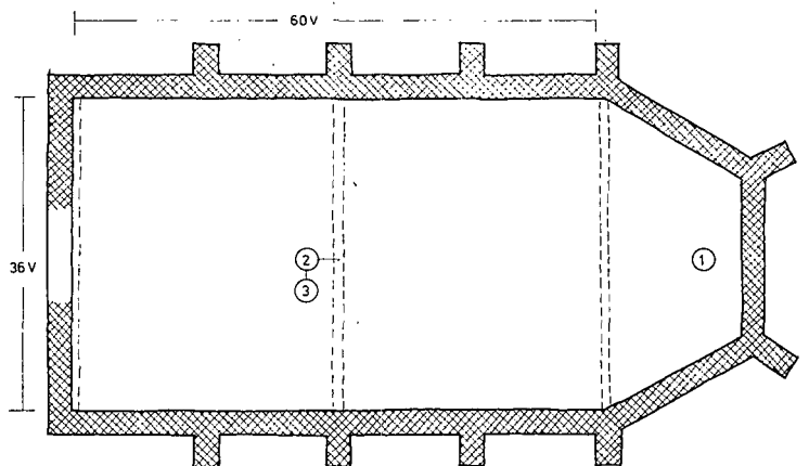
REKONSTRUKTIE PLATTEGROND KAPEL VAN HET GROOT - ZIEKENGASTHUIS TE s-HERTOGENBOSCH. NAAR EEN BESTEK UIT 1487.
