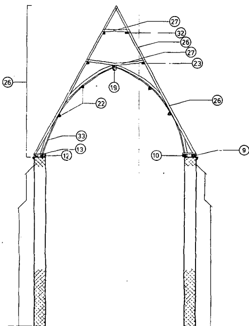
REKONSTRUKTIE DWARSDOORSNEDE VOLGENS EEN BESTEK UIT 1487.
