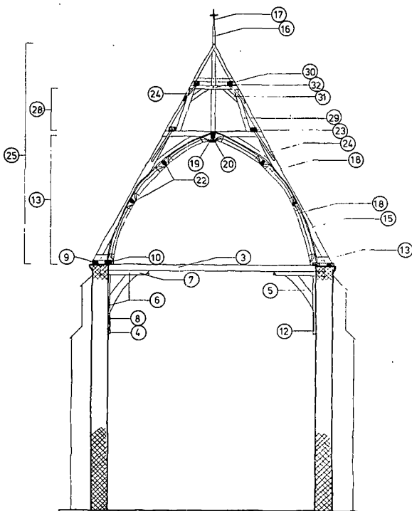
REKONSTRUKTIE DWARSDOORSNEDE VOLGENS EEN BESTEK UIT 1487.
